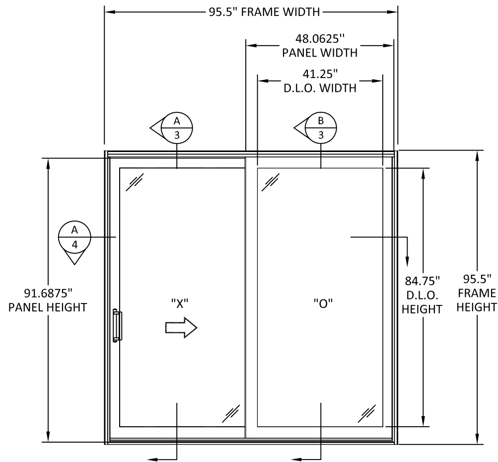
ELEVATION SLIDING DOOR
